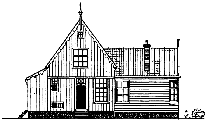
VOORGEVEL
