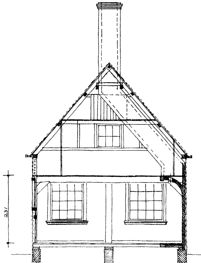
doorsnede CD.
