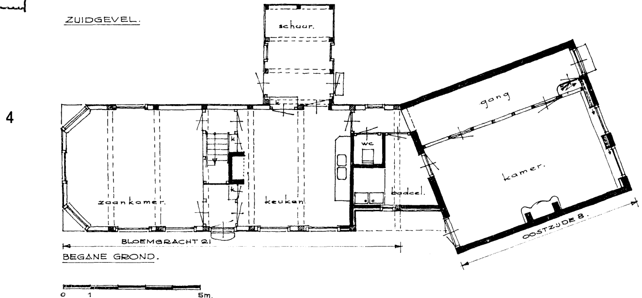
3 en 4: Zijaanzicht en plattegrond van Kalverringdijk 9.
